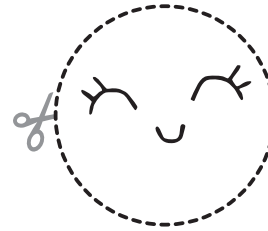
Venus
