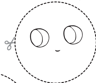
Neptun
