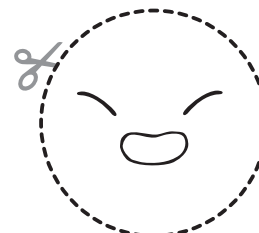
Mars
