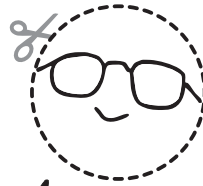
Merkur
