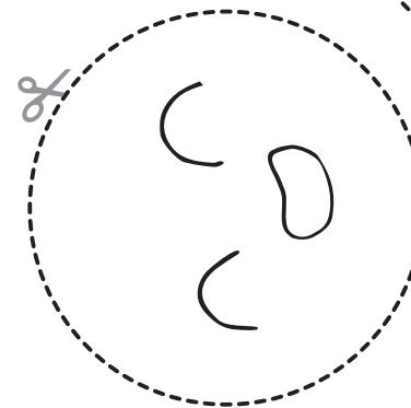
Uranus
