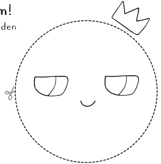
Jupiter
